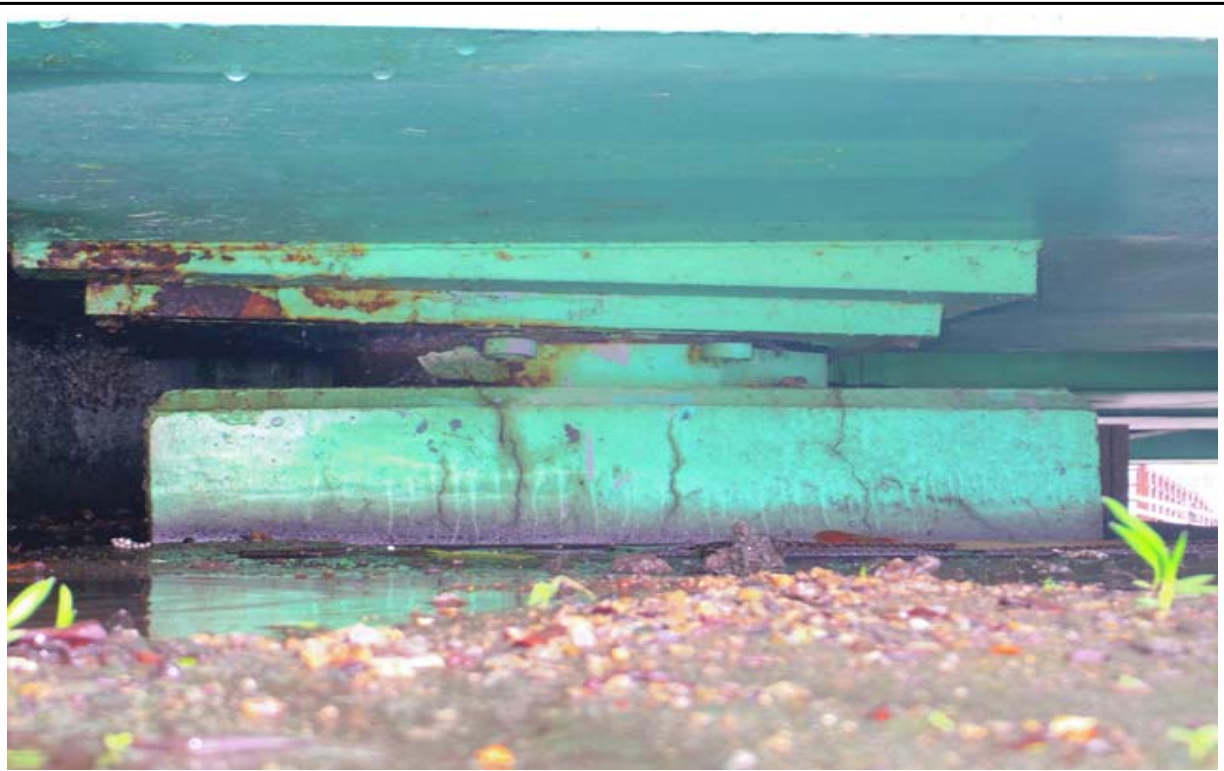
교량받침 균열, 부식(A1-SH2)
