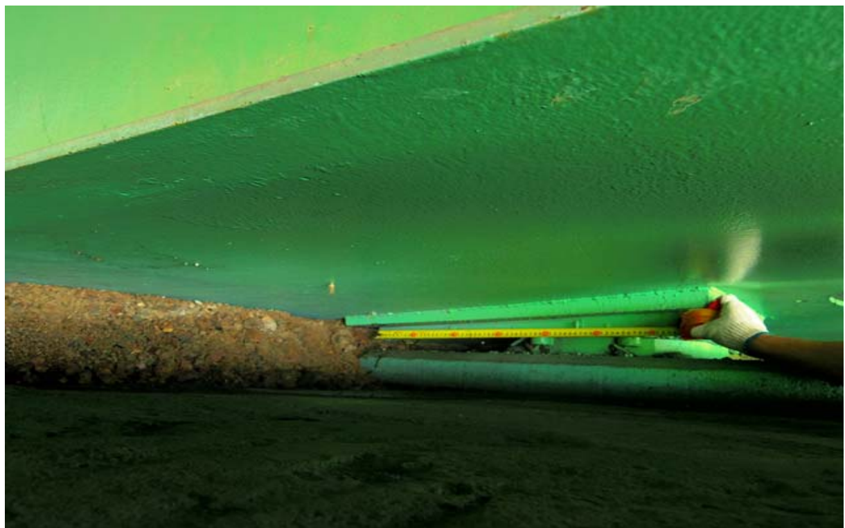
교량받침 A2-SH2(→150mm)
