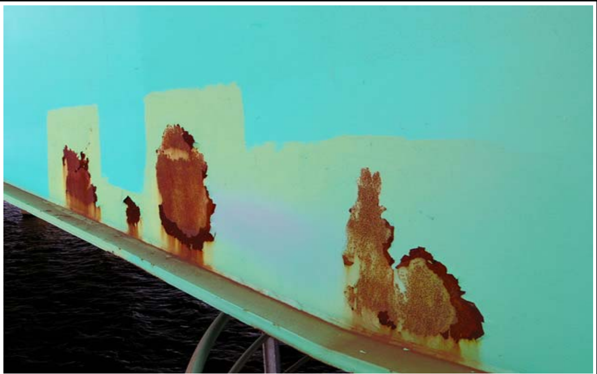
거더외부 부식 (G1-S4)
