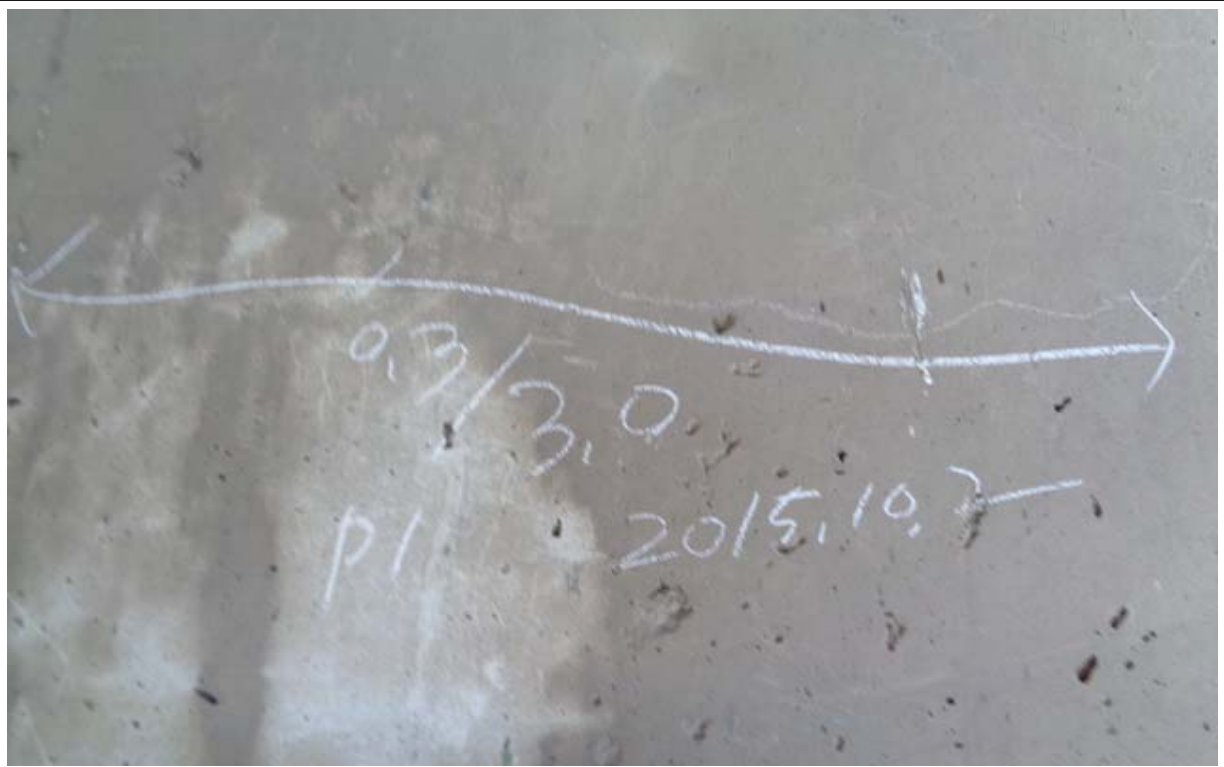
교각 기둥부 균열 (P1)
